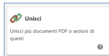
Figura 4 - Unisci PDF
